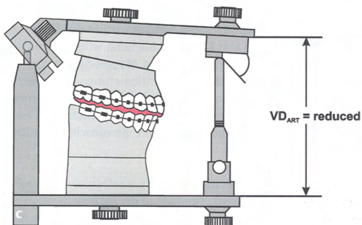
Abb. 10 Herstellung des Zentriksplintes (a). Herstellung der Oberkiefer-Operationssplintes (b). Prinzip der Einstellung des Artikulators für die Herstellung des Postoperationssplintes (c).
