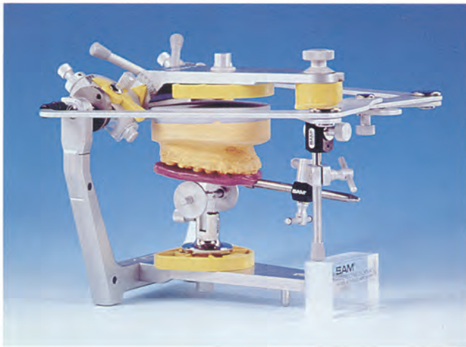
Abb. 4 Modellmontage des Oberkiefers mit Hilfe eines Anatomischen Transferbogens.
