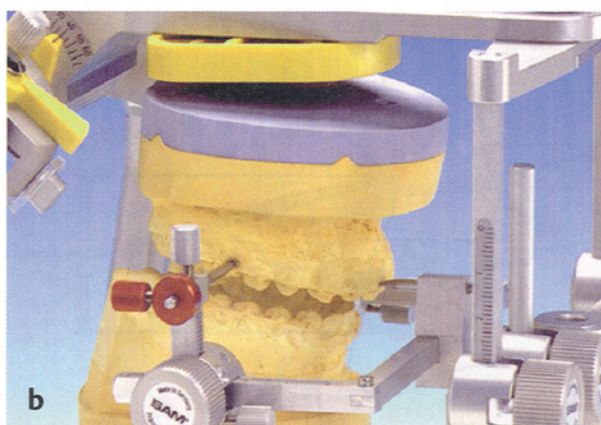
Abb. 9 Modell-Repositionierungs-Instrument in der Ausgangssituation bei der Modelloperation des Oberkiefers (a). Umstellung des zahntragenden Oberkieferkomplexes entsprechend der Planung (b). Situation nach Simulation der Oberkieferoperation (c). Prinzip der Einstellung der Artikulatoren für die Herstellung der Operationssplinte für die Umstellung des Oberkiefers nach dem „3D-Doppelsplint-Verfahren“. Die Stützstiftlänge der beiden Artikulatoren, die die prä- und postoperative Situation repräsentieren, ist jeweils konstant ( VD_{ART} = \text{constant} ).
