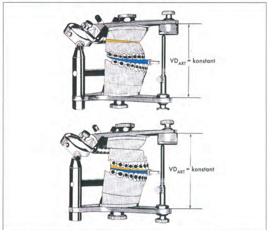
Abb. 19 Prinzip der Einstellung der Artikulatoren für die Herstellung der Operationssplinte zur Umstellung des Oberkiefers nach dem „3D-Doppelsplint-Verfahren“. Die Stützstiftlänge der Artikulatoren, die die prä- und postoperative Situation repräsentieren, ist jeweils konstant ( VD_{ART} = \text{konstant} ).
