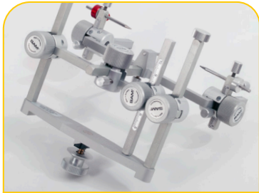
Montage im Artikulatorunterteil Installation in articulator lower part
