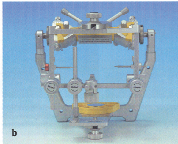
Abb. 7 Ansicht des Modell-Repositionierungs-Instrumentes von der Seite mit den Messspitzen I, II und III; hier montiert am Artikulator SAM 3 (a). Ansicht des Modell-Repositionierungs-Instrumentes von vorn.
